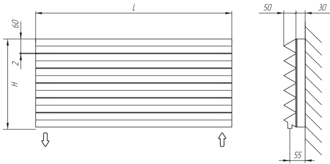
Нижнее подключение
