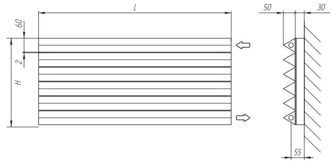
Боковое подключение
